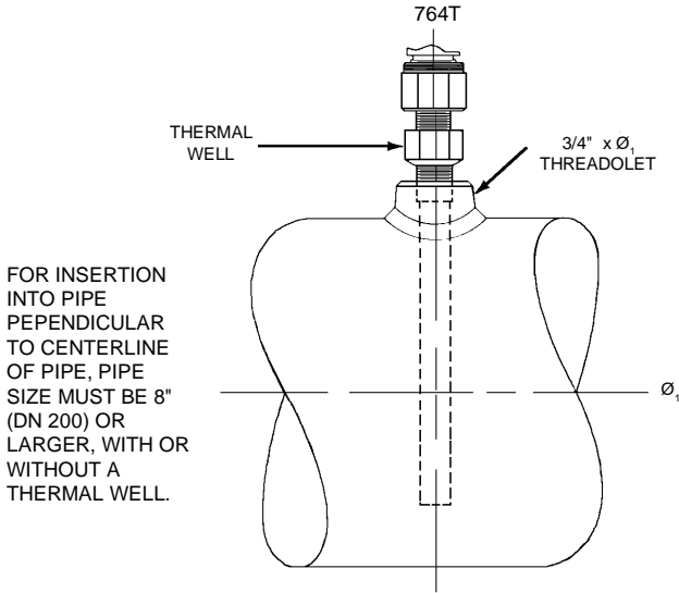
(a): Pipe 8" (DN 200) \phi & Larger
